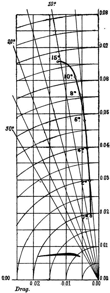
FIG. 3.—Bréguet plane.
